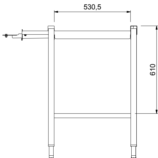
Zepředu
